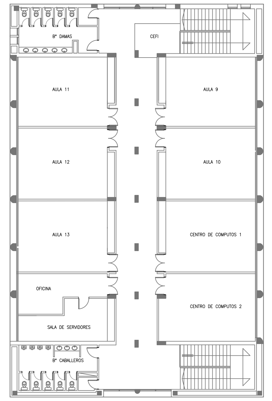
PLANTA ALTA PLANO DE CAÑERÍA EPOXI N° 3
