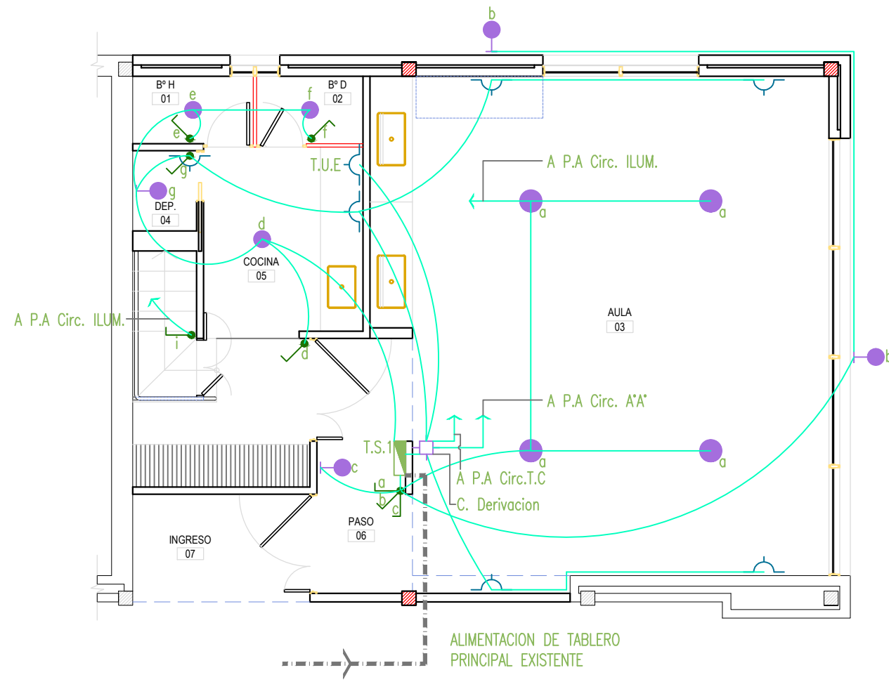
ESQUEMA DE INST. ELECTRICA P.B Esc : 1:75
