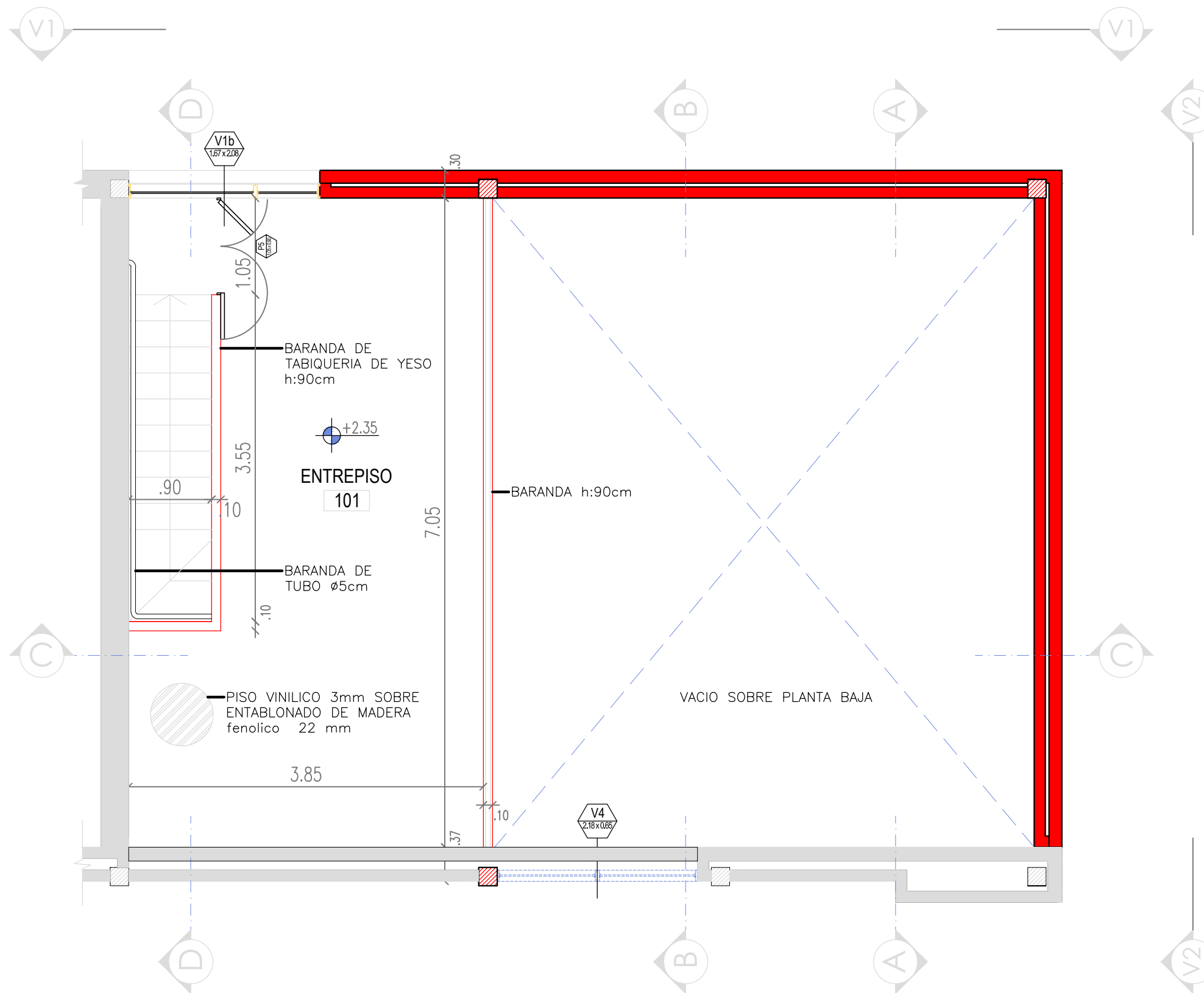
PLANTA DE ENTREPISO Esc : 1:50
