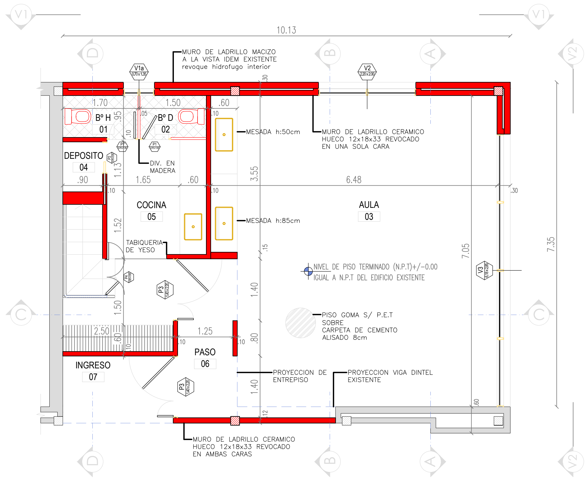
PLANTA BAJA Esc : 1:50
